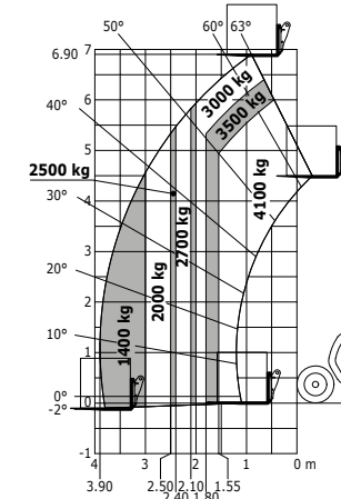
All terrain load chart (EN 1459 B)
