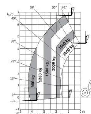
All terrain load chart (EN 1459 B)
